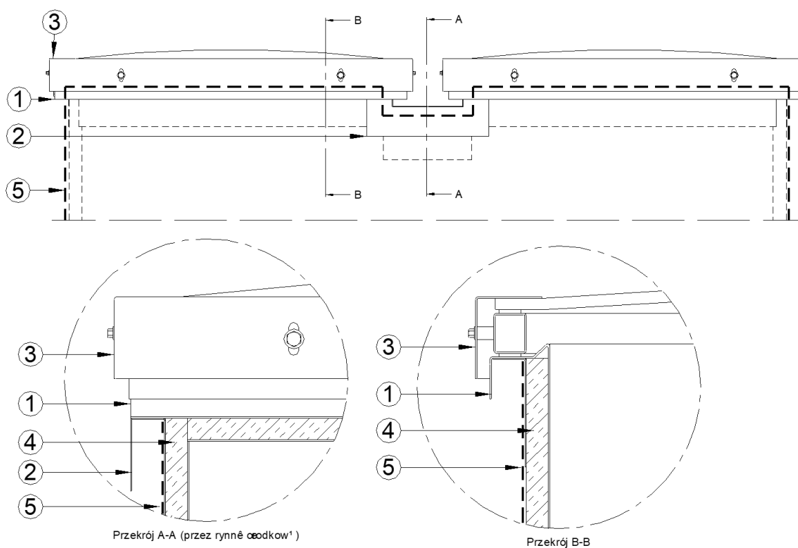
Rys. 14 Schemat montażu izolacji przeciwwodnej w klapie mcr PROLIGHT.
