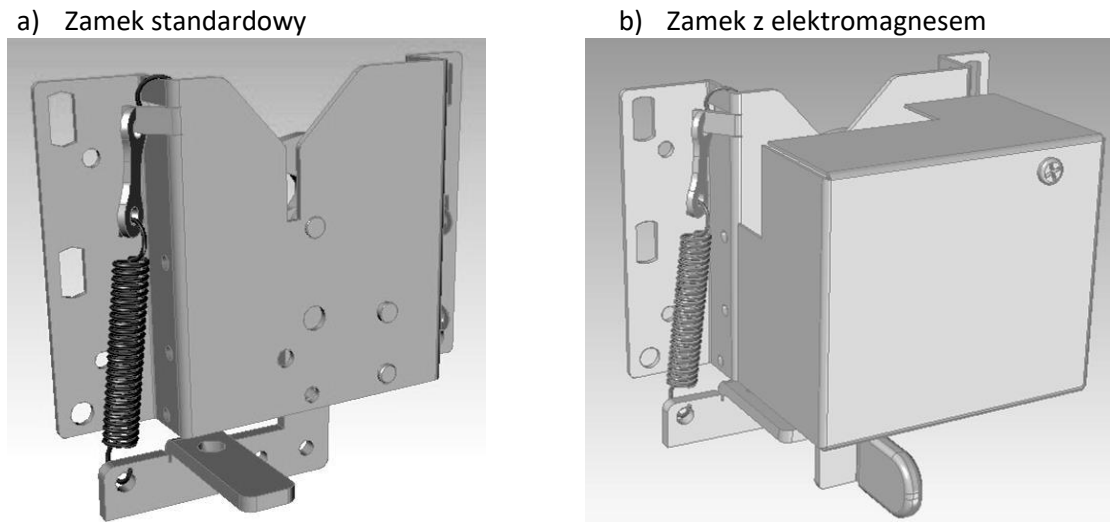
Rys. 38 Typy zamków dla sterowania mechanicznego.
