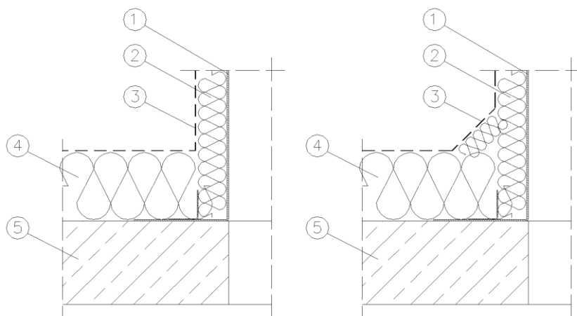
detale B
