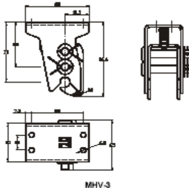
Rys. 22 Konsola hakowa.
