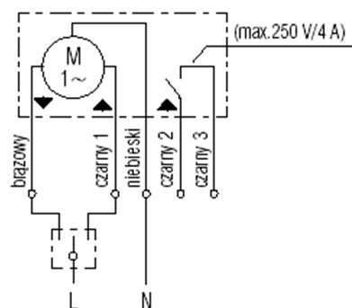
Rys. 37 Siłownik JMBB-500-300-LA.
